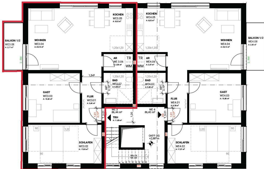
12 Grundriss Whg. 3
