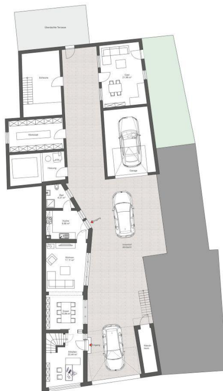
EG
